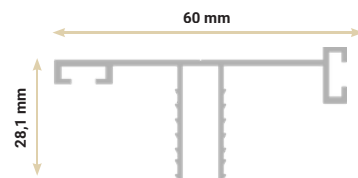
6 Cliquet latéral Side clip
