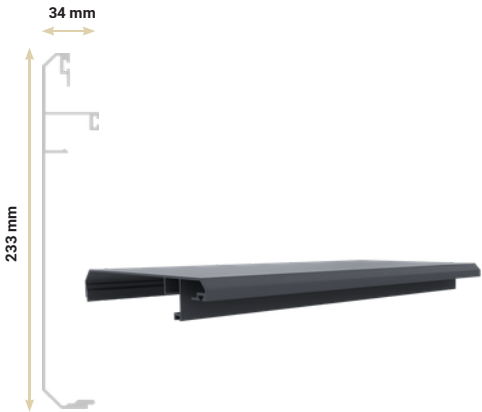
1 Capot supérieur Top cover
