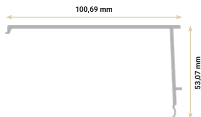
8 Cliquet décoratif profil mural Clips for decorative wall profile
