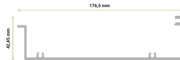
12 Chéneau droit Right gutter
