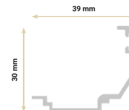
12 Profil pour encadrement de panneau Panel framing profile
