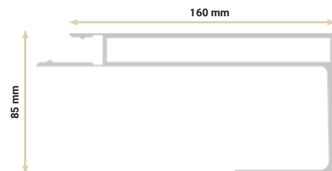
6 Capot de profil de faîtage Ridge profile cover
