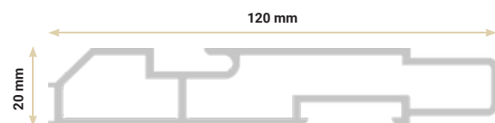
8 Profil de capot de poutre Ridge profile cover
