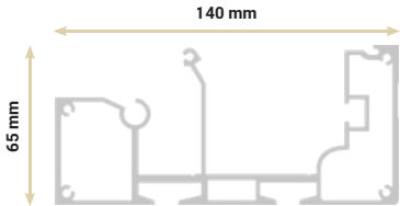
6 Barre de charge Charge Bar
