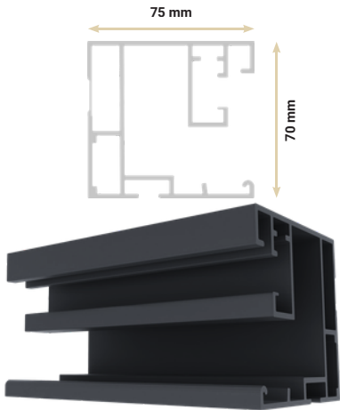
2 Guidage latéral Lateral Guidance
