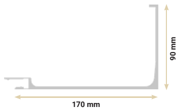
7 Capot de profil de poutre Ridge profile cover
