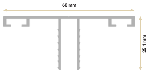
5 Cliquet supérieur Top clip
