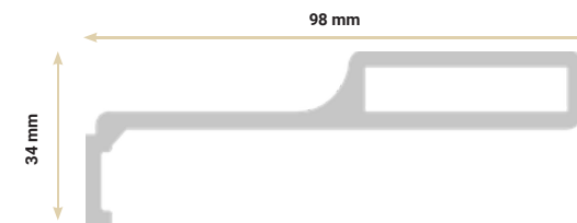
10 Profil d'entraînement Drive Profile
