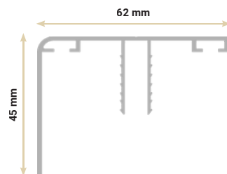
6 Clip de fixation chevron d'extrémité Side clip
